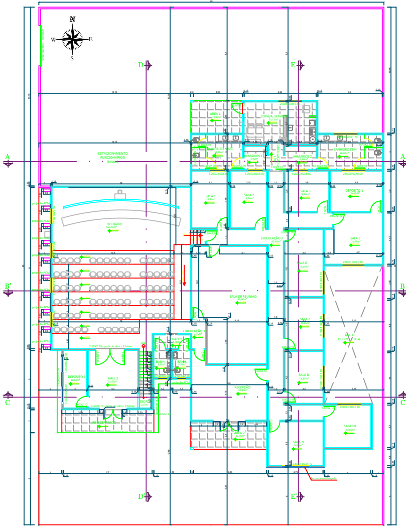
PLANTA BAIXA
