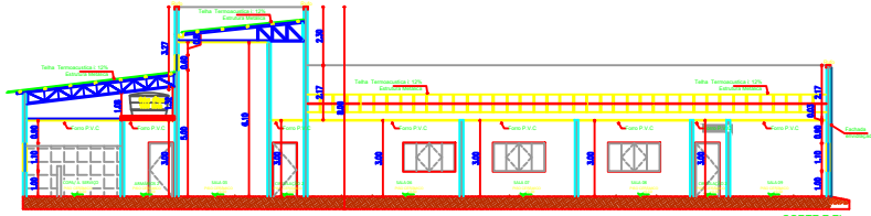
CORTE E-E
