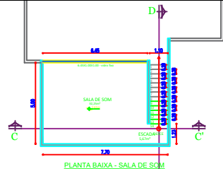
PLANTA BAIXA - SALA DE SOM
