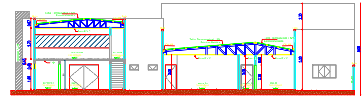
CORTE C-C''
