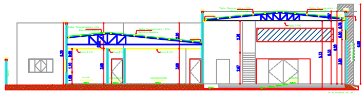
CORTE B-B''
